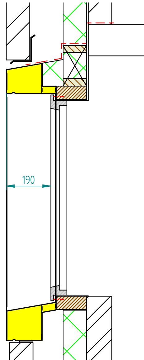
Doorsnede A-A
